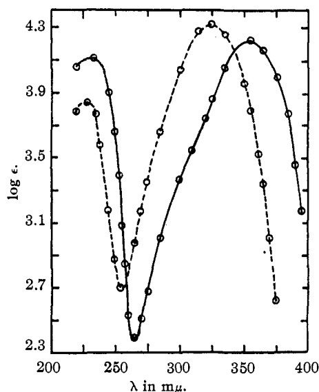
Fig. 1.— ---, Acetylacetone anil; —, 3-acetyl-1,4-dihydroquinoline.
