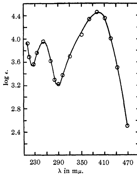
Fig. 3.— p -Dimethylaminobenzalacetone.
